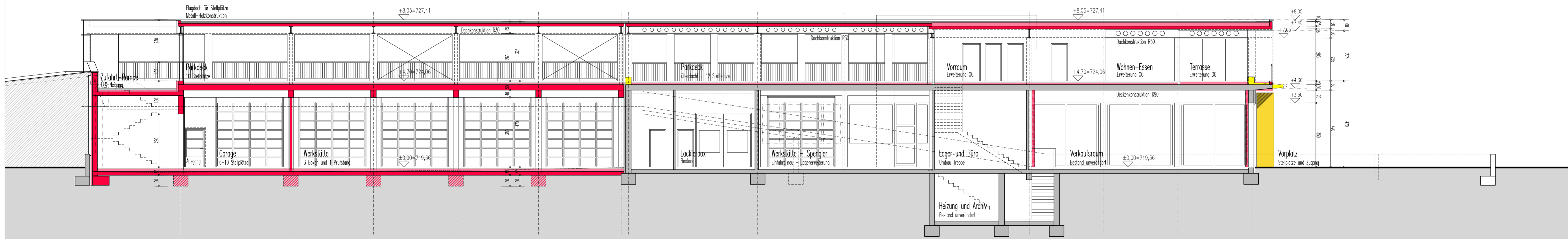
SCHNITT S1 M1:100
