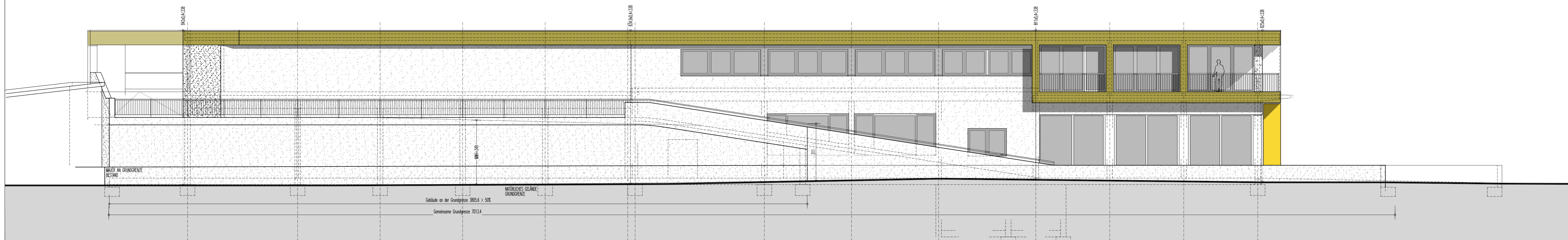
ANSICHT WEST M1:100
